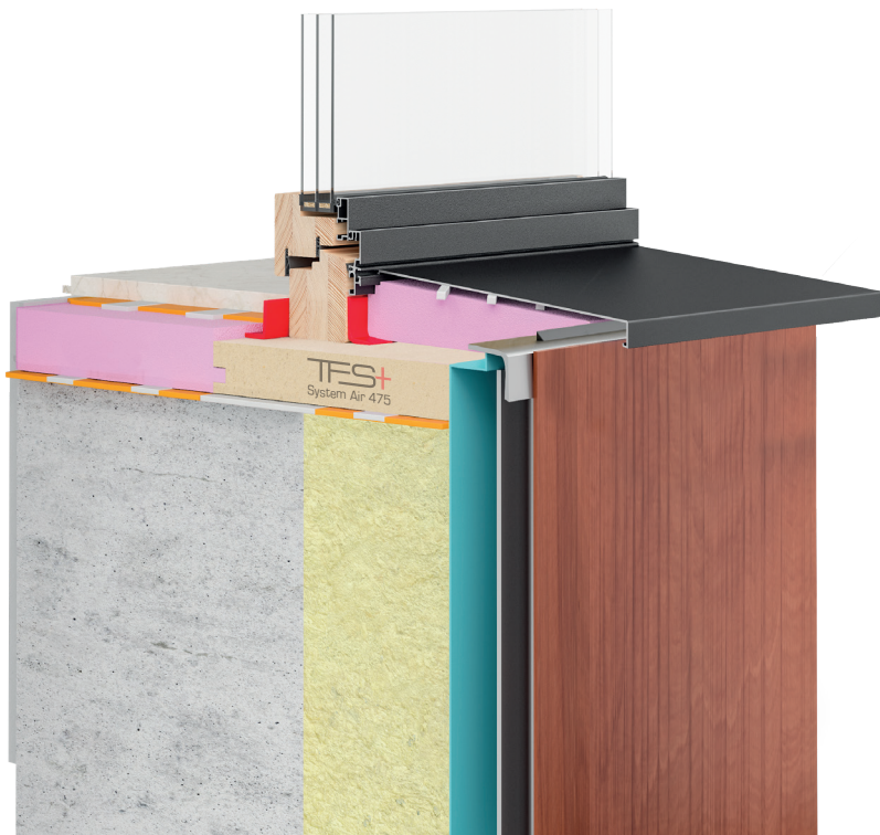
System Air 475 Dicke 50/40 mm Für hinterlüftete Fassade
