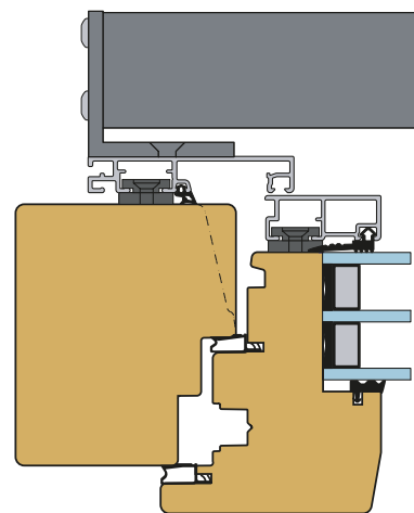
L-MONTAGE
