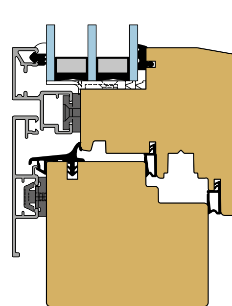
GS ECO 400 Detailschnitt
