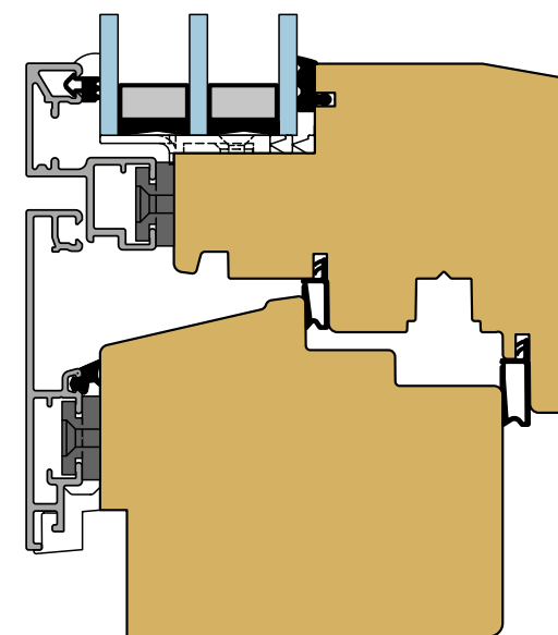
GS STRATOS 400 Detailschnitt
