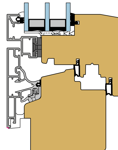
GS PREMIUM 400 Detailschnitt
