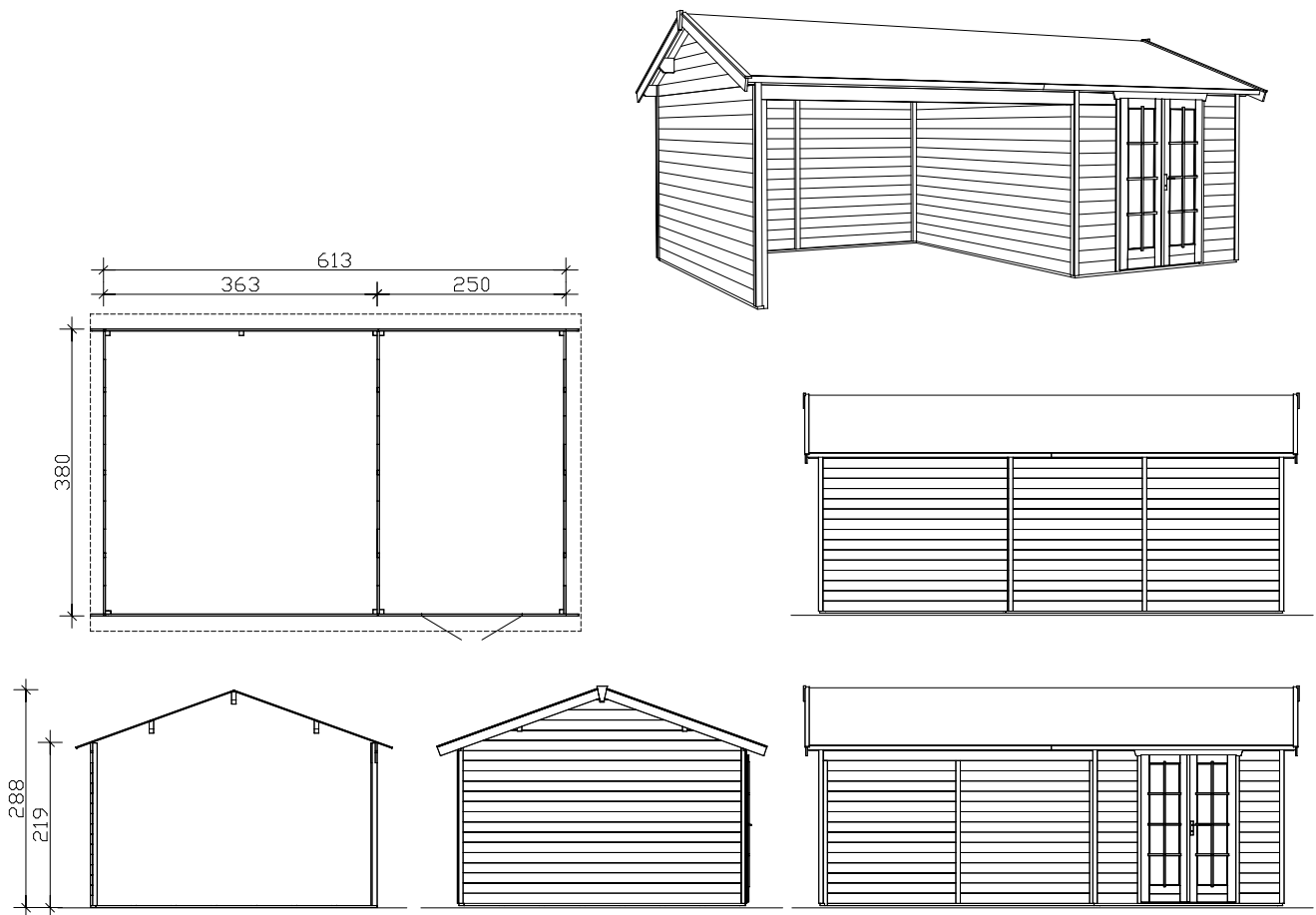
Põhiplaan, lõige ja vaated M 1:100
