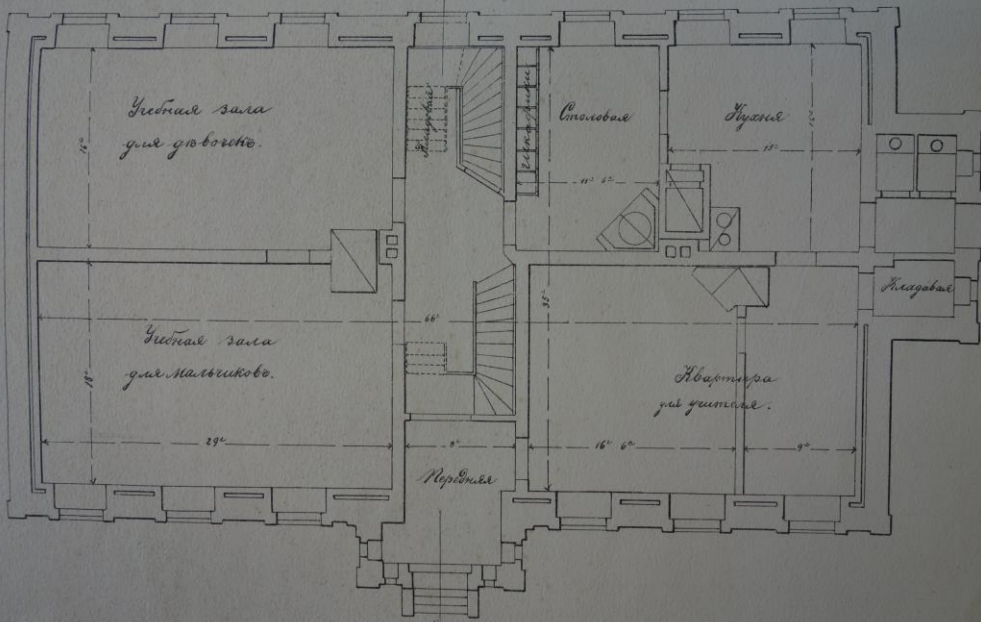
Угловой план.
