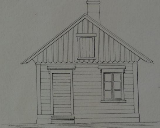
Боковой фасад.
