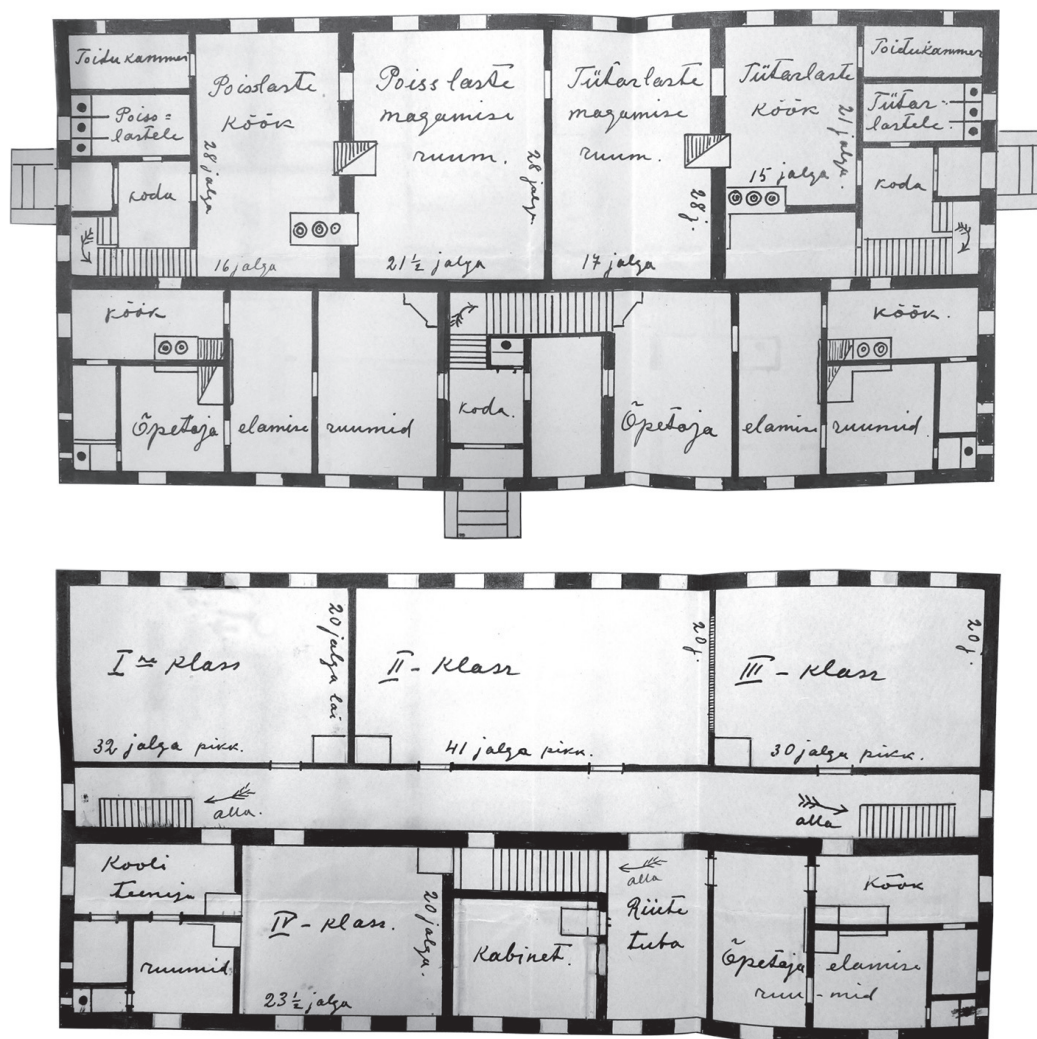
Raikküla koolimaja I ja II korruse põhiplaan, 1908. Ehitusmeister Juhan Valdes. TLA.884.4.1096.
