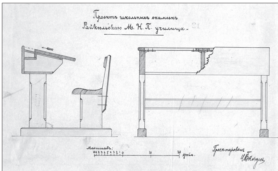
Raikküla koolile kavandatud klassipink. Juhan Valdese joonistus 1909. aastast. RA, EAA.3079.1.301. Samad pingid olid koolis kasutusel vähemalt 1960. aastateni.
