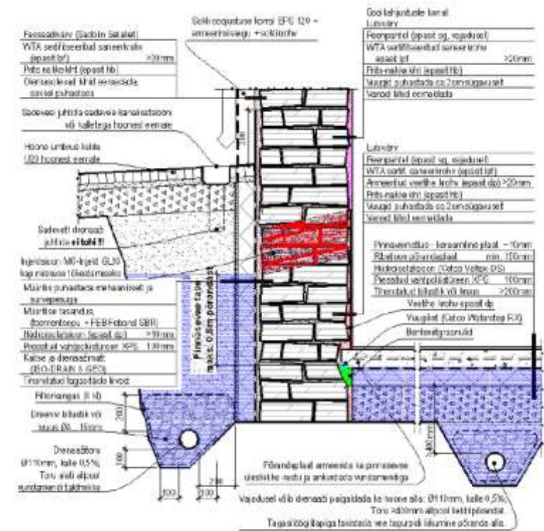
Joonis 13.8 Keldri veetõke muutuva (võib tõusta kuni 0,5 m keldri põrandapinnast) pinnasevee taseme korral.
