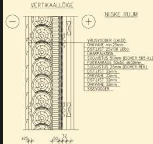
Joonis 3. Palkmajasauna sein
