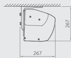
Kinnitus katusele
