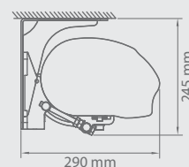
Kinnitus katusele
