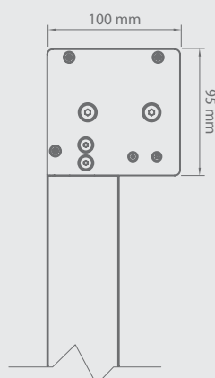
Kasetti mõõdud
