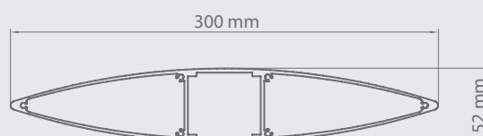
Ribade lõik
