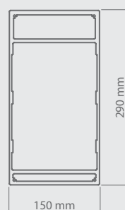
Tala lõik
