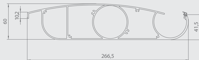
Posti lõik
