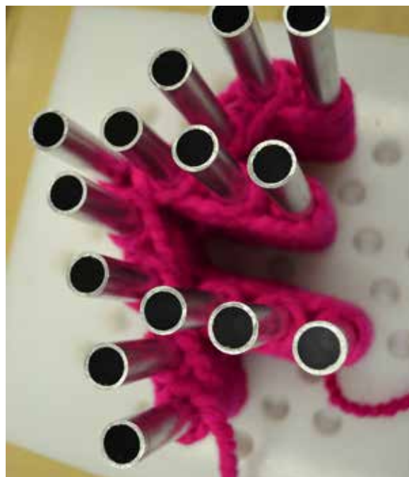
MultiWeave põhimõte on laadida lõimelõngad torukestesse ja siis nende torukeste ümber jooksutada etteprogrammeeritud viisil koelõnga. Kui asi tehtud, eemaldatakse tugikonstruktsioon ja tulemuseks ongi 3Dprinditud ruumiline tekstiil.
