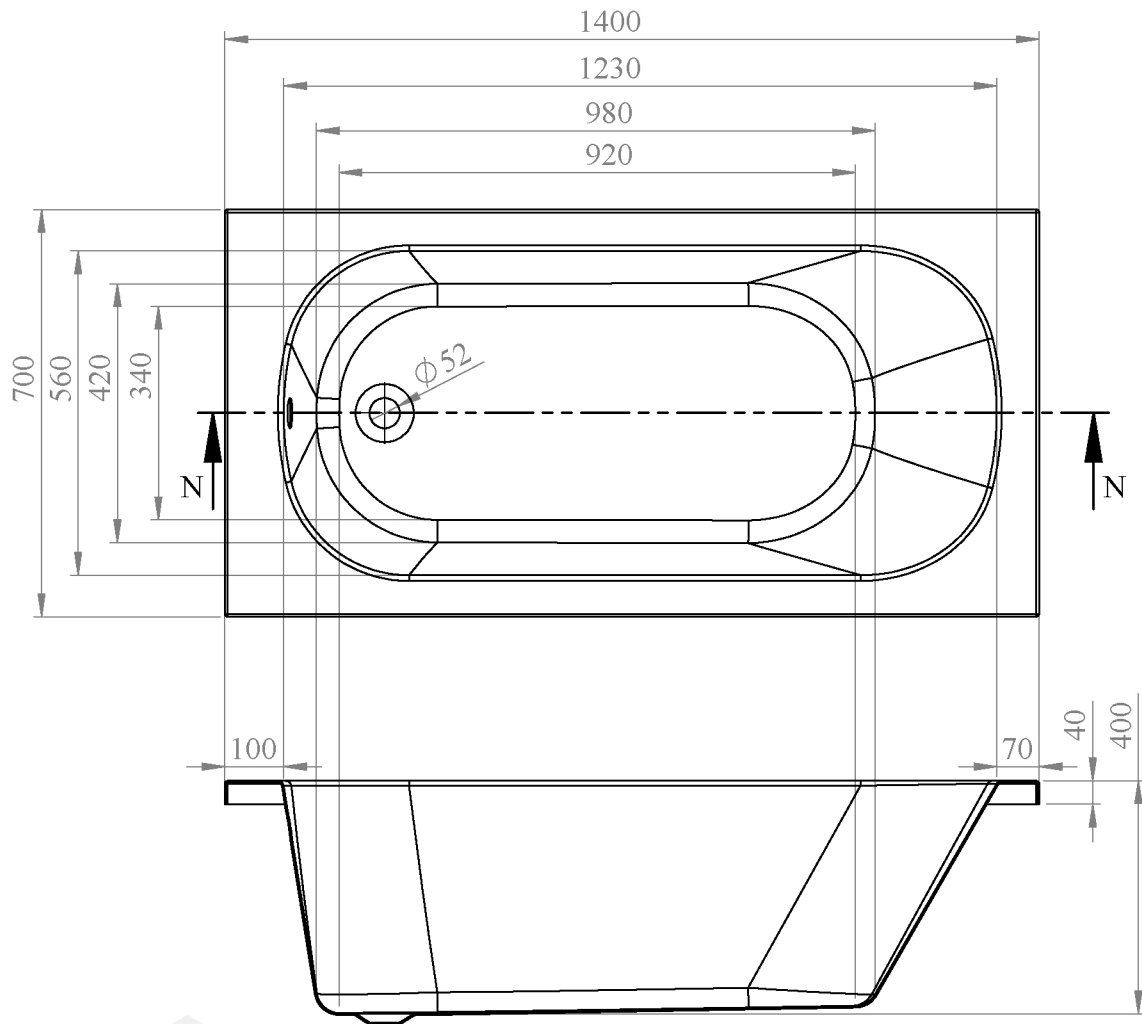
PRZEKRÓJ N-N SKALA 1 : 13
