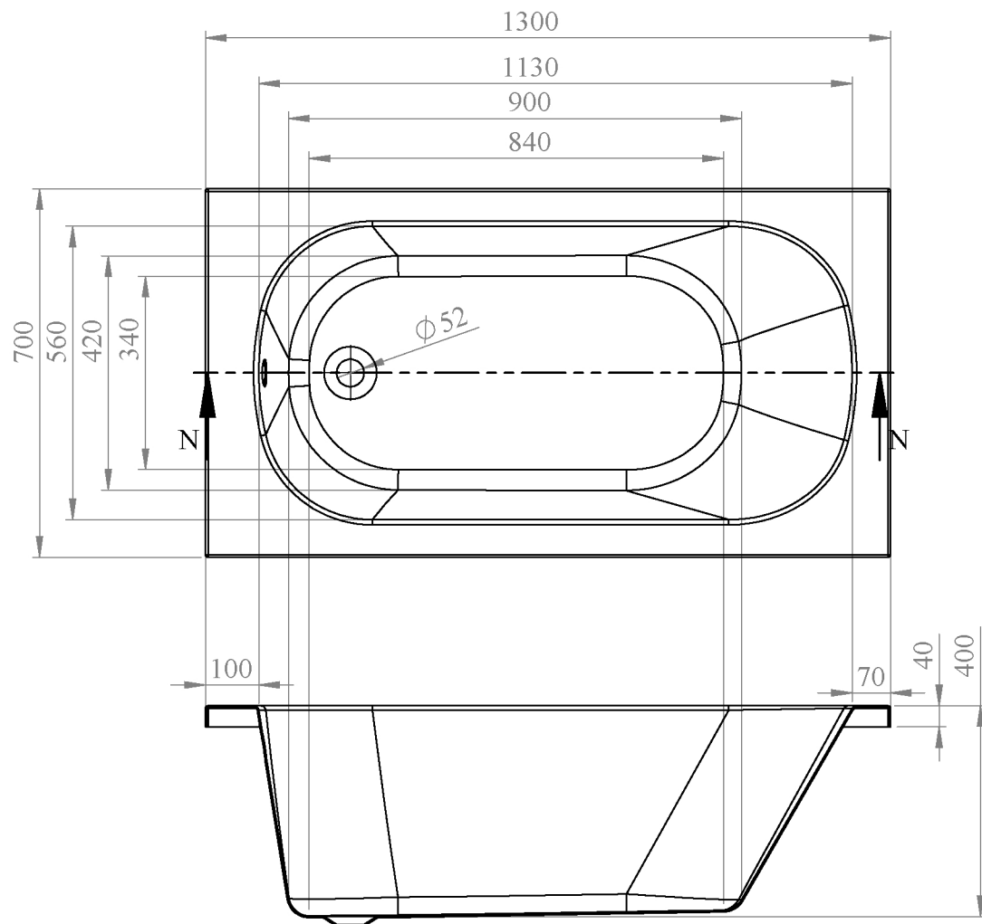
PRZEKRÓJ N-N SKALA 1 : 13
