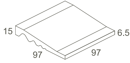
Duř parçası Shower inclined end edge M 10 x 10 cm / 4" x 4" 97 x 97 x 6.5 / 15 mm EN14411 Bla
