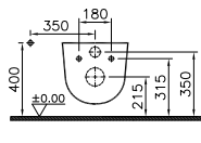
Standard connection Standart bağlantı
