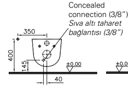
Concealed connection Sıva altı bağlantı
