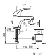
Monocomando lavabo Single lever washbasin mixer Jednopáková umyvadlová baterie
