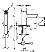
Monocomando ad incasso per bidé WC Canna girevole e Flessibile satin
