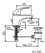
Monocomando lavabo ecologico Single lever washbasin mixer ecological Jednopáková umyvadlová baterie s ekologickou funkcí
