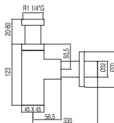
Sifone telescopico a vista per lavabo Telescopic visible basin drain trap Čtverhranný, výsuvný umyvadlový sifon viditelný
