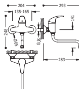
Monocomando a muro Single lever wall sink mixer Jednopáková dřezová baterie nástěnná
