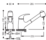
Monocomando lavello verticale estraibile (2 funzioni) Single lever single hole sink mixer with removable spout (2 operations) Jednopáková dřezová baterie svislá s vyjímatelnou sprškou (2 funkce)
