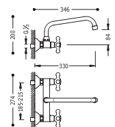
Gruppo lavello parete Distanza da parete di 330 mm. Wall sink mixer Distance from wall 330 mm. Nástěnný dřezový kuchyňský set vzdálenost od zdi 330 mm
