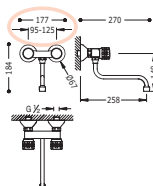
Gruppo lavello parete Distanza da parete di 260 mm.
