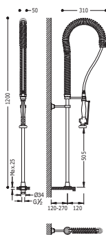
Monocomando lavello verticale Single lever single hole sink mixer Dřezová kuchyňská baterie
