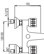
Gruppo vasca Doccetta anticalcare con supporto orientabile. Flessibile doppia graffatura
