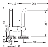
Monocomando lavello verticale Single lever single hole sink mixer Jednopáková dřezová kuchyňská baterie
