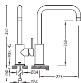
Monocomando lavello verticale Single lever single hole sink mixer Jednopáková dřezová kuchyňská baterie
