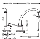
Monocomando lavello verticale Single lever single hole sink mixer Jednopáková dřezová baterie svislá
