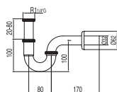
Sifone curvo articolato per lavabo Curved, articulated drain trap for basin Umyvadlový sifon s kloubovým zakřivením
