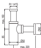
Sifone telescopico a vista per lavabo Telescopic visible basin drain trap Výsuvný umyvadlový viditelný sifon
