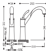
Monocomando lavello verticale Single lever single hole sink mixer Jednopáková dřezová baterie svislá
