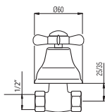
Rubinetto di arresto filettato 1/2" Valve 1/2" Uzavírací ventil 1/2"
