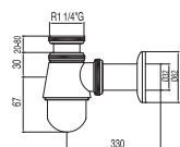
Sifone a bottiglia facilmente ispezionabile per bidet Self-inspecting bottle-type drain trap for bidet Bidetový lahvový sifon, rozšroubovatelný
