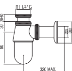
Sifone a bottiglia facilmente ispezionabile per lavabo Self-inspecting bottle-type drain trap for basin Umyvadlový lahvový sifon, rozšroubovatelný
