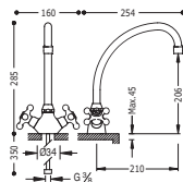
Monoblocco lavello verticale Single hole sink mixer Dvoupáková dřezová kuchyňská baterie
