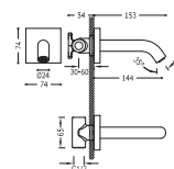
Canna parete Wall spout Nástěnné ramínko
