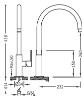
Monocomando lavello verticale Single lever single hole sink mixer Jednopláková dřezová kuchyňská baterie
