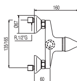
Monocomando doccia Doccetta anticalcare con supporto orientabile. Flessibile doppia graffatura Single lever shower mixer Anti-limescale hand shower with directable support. Double interlocked shower hose
