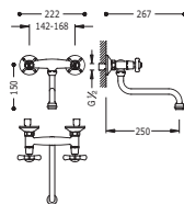
Gruppo lavello parete Distanza da parete di 250 mm. Wall sink mixer Distance from wall 250 mm. Nástěnný dřezový kuchyňský set vzdálenost od zdi 250 mm
