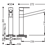
Monocomando lavello verticale canna lunga Single lever single hole sink mixer tube spout Jednopáková dřezová kuchyňská baterie dlouhé ramínko
