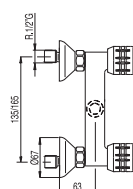
Gruppo doccia Doccetta anticalcare con supporto orientabile. Flessibile doppia graffatura
