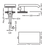
Erogatore a cascata Cascade cast spout Ramínko s vodopádem
