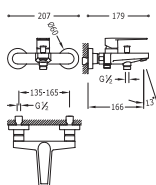
Monocomando vasca Doccetta anticalcare (299.631.08) con supporto orientabile. Flessibile satin (91.34.609).
