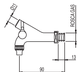
Rubinetto vino N° 1/N Wine tap N° 1/N Kohoutek na víno č. 1/N
