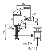
Monocomando bidet Single lever bidet mixer Jednopáková bidetová baterie
