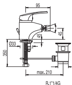
Monocomando bidé Single lever bidet mixer Jednopáková bidetová baterie
