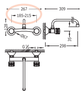
Gruppo lavello parete Wall sink mixer Nástěnný dřezový celek
