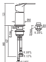
Monocomando bidet con doccetta Bidet mixer tap with small shower head Jednopáková bidetová baterie se sprškou
