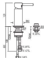
Monocomando bidet con doccetta Bidet mixer tap with small shower head Jednopáková bidetová baterie se sprškou
