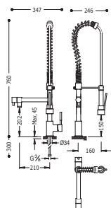
Monocomando lavello verticale Single lever single hole sink mixer Jednopáková dřezová kuchyňská baterie
