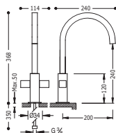
CUCINA DOPPIO COMANDO / DUAL-CONTROL KITCHEN TAPS / DŘEZOVÉ BATERIE S DVOUPÁKOVÝM MECHANISMEM
