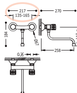
Gruppo lavello parete Wall sink mixer Nástěnný dřezový celek
