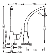
Monocomando lavello verticale Single lever single hole sink mixer Jednopáková dřezová baterie svíslá
