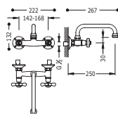
Gruppo lavello parete Distanza da parete di 250 mm. Wall sink mixer Distance from wall 250 mm. Nástěnný dřezový kuchyňský set vzdálenost od zdi 250 mm
