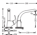
Monocomando lavello verticale Single lever single hole sink mixer Jednopáková dřezová baterie svíslá
