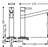
Monocomando lavello verticale canna lunga Single lever single hole sink mixer tube spout Jednopáková dřezová kuchyňská baterie dlouhé ramínko
