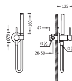
Monocomando ad incasso per bidé WC Supporto a destra o a sinistra, intercambiabile. Flesso satinato. * Opzione Cartongesso
