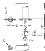
Monocomando bidet con doccetta Bidet mixer tap with small shower head Jednopáková bidetová baterie se sprškou
