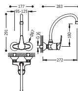
Monocomando a muro Single lever wall sink mixer Jednopáková dřezová baterie nástěnná
