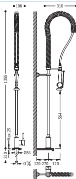
Monocomando lavello verticale Single lever single hole sink mixer Jednopáková dřezová kuchyňská baterie
