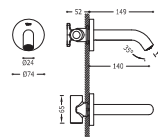
Canna parete Wall spout Nástěnné ramínko
