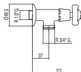
Rubinetto lavatrice 3/4" Avvitare Washing machine tap 3/4" Kohoutek pro pračku Výstup - závit 3/4"
