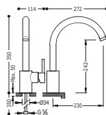
Monocomando lavello verticale Single lever single hole sink mixer Jednopáková dřezová kuchyňská baterie
