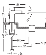
Monocomando bidet Single lever bidet mixer Jednopáková bidetová baterie
