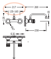
Gruppo lavello parete Wall sink mixer Nástěnný dřezový celek
