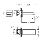
Erogatore a cascata Cascade cast spout Ramínko s vodopádem
