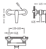
Monocomando doccia Doccetta anticalcare (299.631.08) con supporto orientabile. Flessibile satin (91.34.609.15).
