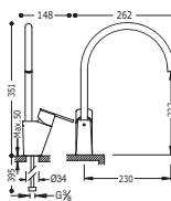
Monocomando lavello verticale Single lever single hole sink mixer Jednopáková dřezová kuchyňská baterie
