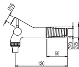
Rubinetto vino N° 2/C Wine tap N° 2/C Kohoutek na víno č. 2/C
