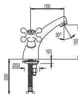
Monoblocco lavabo Single hole wash-basin mixer Dvoupáková umyvadlová baterie
