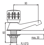
Monoblocco lavabo Basin pillar tap Umyvadlová baterie
