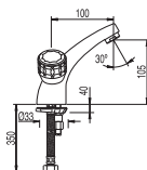
Monoblocco lavabo Basin pillar tap Umyvadlová baterie
