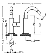
Single lever bidet mixer Monocomando bidet Jednopláková bidetová baterie
