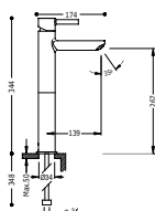
Single lever washbasin mixer with base extension Monocomando lavabo con prolunga inferiore Jednopáková umyvadlová baterie s nástavcem
