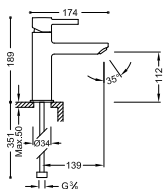
Single lever washbasin mixer Monocomando lavabo Jednopáková umyvadlová baterie
