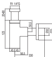
Telescopic visible basin drain trap Sifone telescopico a vista per lavabo Čtverhranný, výsuvný umyvadlový sifon viditelný
