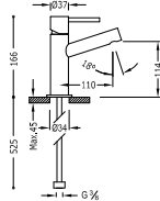
Single lever washbasin mixer Monocomando lavabo Jednopláková umyvadlová baterie
