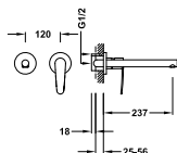
Monomando a muro Corpo a incasso indivisibile con smorzatori. Guarnizione antiumidità. Canna 237 mm.
