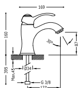
Single lever washbasin mixer Monocomando lavabo Jednopáková umyvadlová baterie
