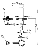
Bidet mixer tap with small shower head Monocomando bidet con doccia Jednopláková bidetová baterie se sprškou
