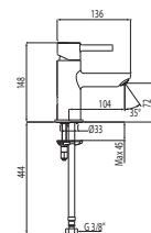
Single lever washbasin mixer Monocomando lavabo Jednopáková umyvadlová baterie
