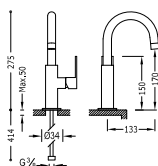
Single lever washbasin mixer Monocomando lavabo Jednopáková umyvadlová baterie
