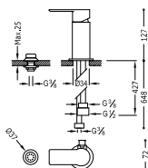
Bidet mixer tap with small shower head Monocomando bidet con doccetta Jednopláková bidetová baterie se sprškou
