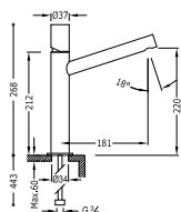
Single lever washbasin mixer long spout Monocomando lavabo canna lunga Jednopláková umyvadlová baterie dlouhé ramínko
