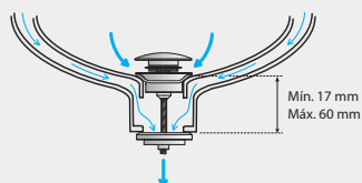
Counter top with overflow drain Piano con troppopieno Deska s přepadem
