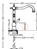
Single hole sink mixer FOLDING Monocomando lavello verticale ABBATTIBILE Jednopávková dřezová kuchyňská baterie SKLOPNÁ
