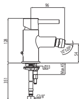
Single lever bidet mixer Monocomando bidet Jednopáková bidetová baterie
