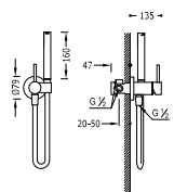
Concealed single lever bidet/toilets Left or right support, interchangeable. Sateen hose. Monocomando ad incasso per bidè WC Supporto a destra o a sinistra, intercambiabile. Flesso satinato. Jednopávková podomítková baterie pro bidet WC Výmennitelný držák zprava či zleva. Sprchová mosazná baterie s omezovacím hrdlem 5 l/m. Systém proti kapání a flex hadice SATIN
