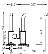
Single lever single hole sink mixer Monocomando lavello verticale Jednopáková dřezová kuchyňská baterie
