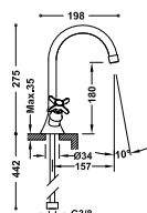
Single hole wash-basin mixer Monoblocco lavabo Dvoupáková umyvadlová baterie
