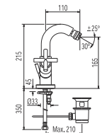
Single hole bidet mixer Monoblocco bidet Dvoupáková bidetová baterie
