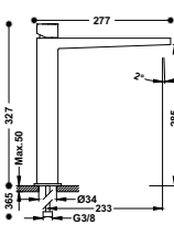
Single lever washbasin mixer Monocomando lavabo Jednopáková umyvadlová baterie
