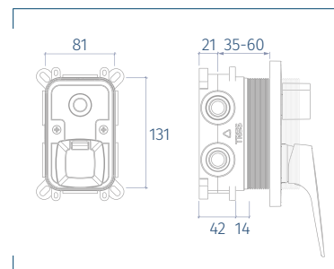
Installation dimensions Livelli di installazione Montážní kóty
