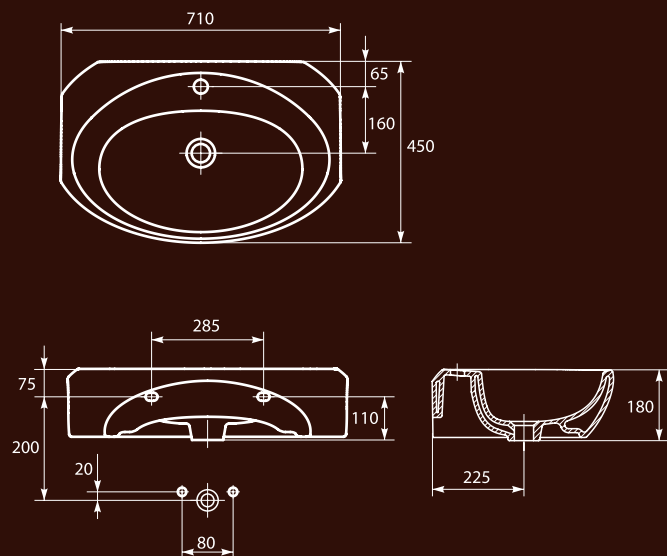
Umywalka BILBAO 70
