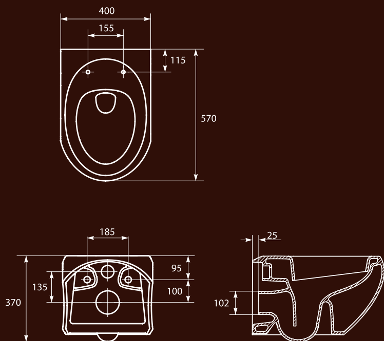
Miska zawieszana BILBAO
