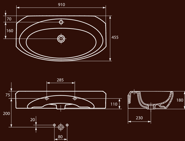
Umywalka BILBAO 90
