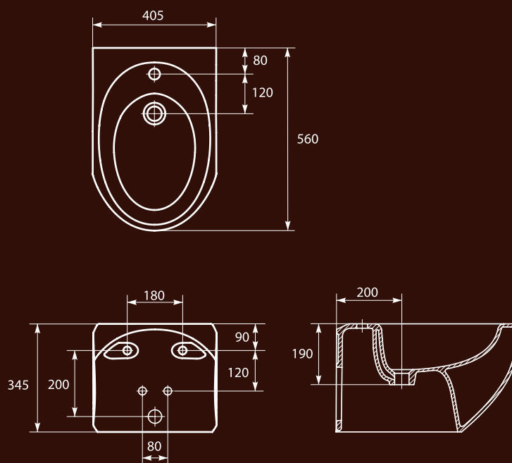
Bidet zawieszany BILBAO
