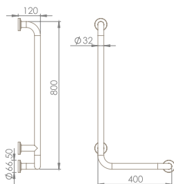
L Type Grab Bar 9AD0800030
