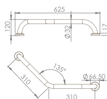
Angled Grab Bar 9AD0310030
