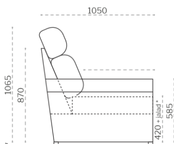
külgvaade
