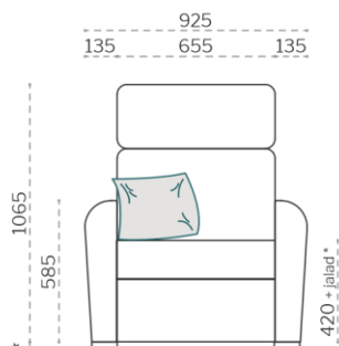
eestvaade
