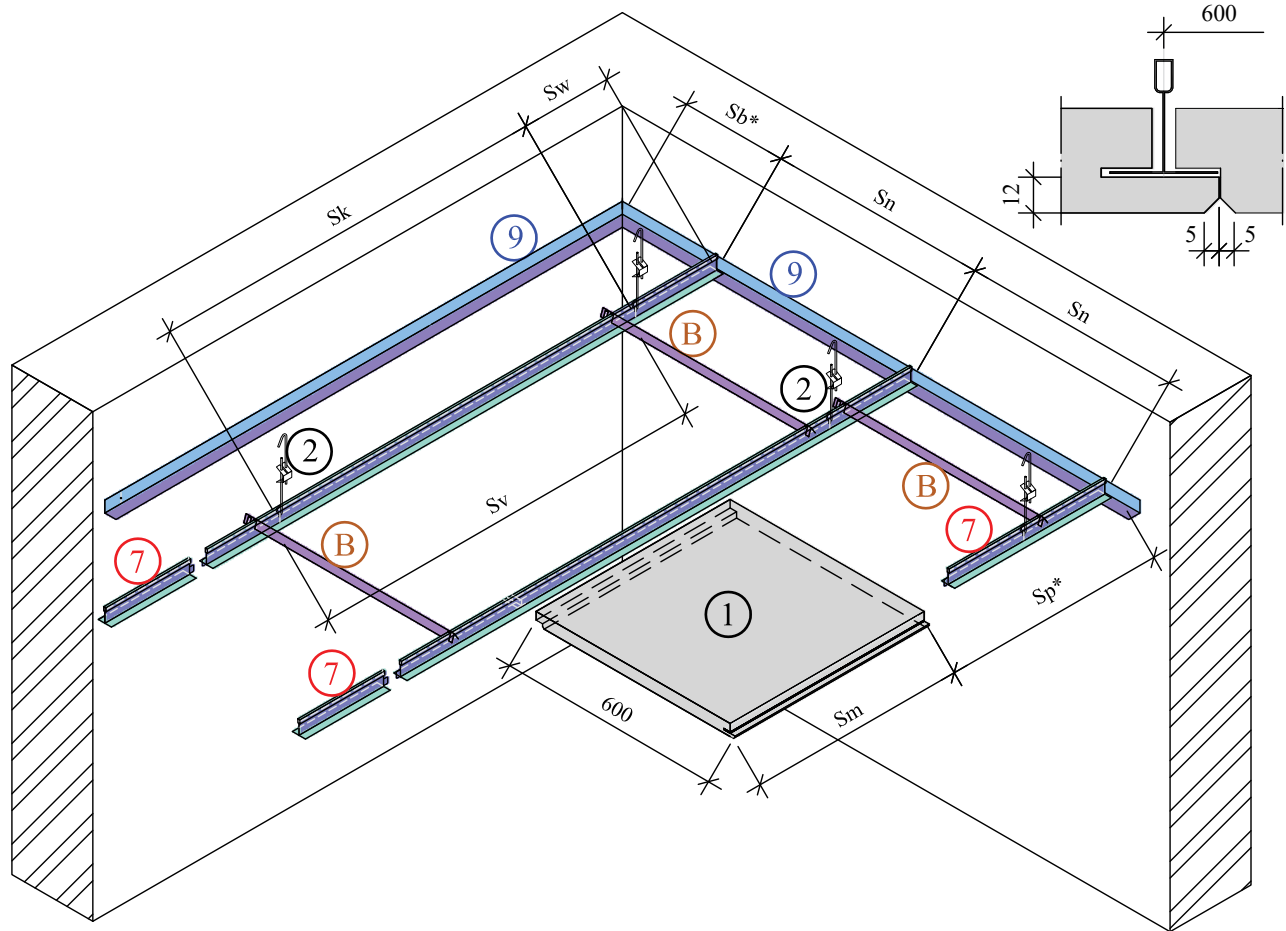
Abb. 7.2: T-Profilrahmen
