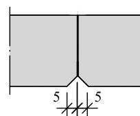
Kantenprofil von CEWOOD Akustikplatten P5
