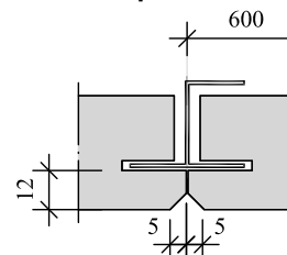
Kantenprofil von CEWOOD Akustikplatten P5H
