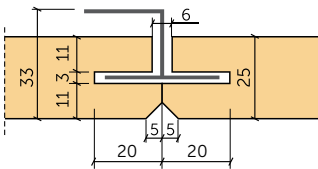
Plattendicke: 25 mm
