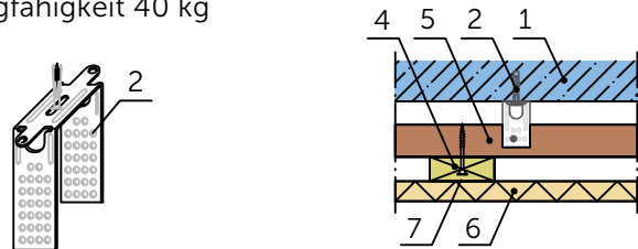
Stoß zwischen Längskanten
