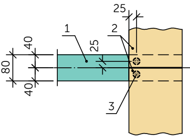
Platte 1200 x 600 mm, längs mit 6 Schrauben befestigt
