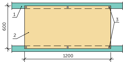
Platte 1200 x 600 mm, längs mit 6 Schrauben befestigt
