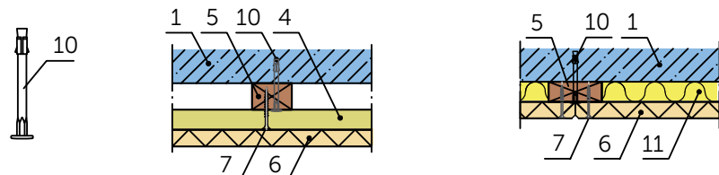
Zweilagige Unterkonstruktion
