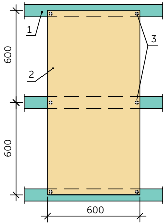
Platte 1200 x 600 mm, mit 6 Schrauben befestigt
