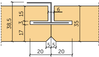
Plattendicke: 35 mm
