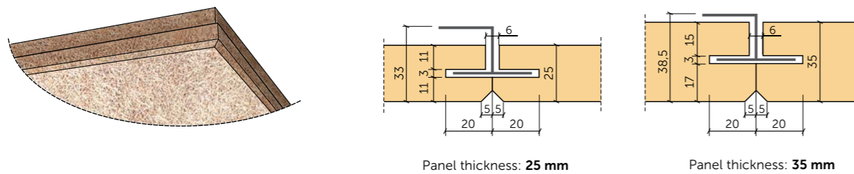
CEWOOD clips
