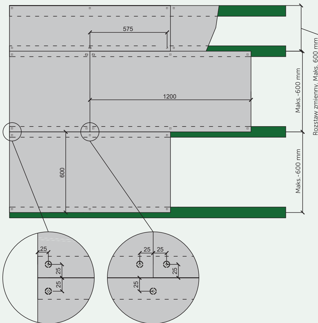
Schemat rozmieszczenia wkrętów
