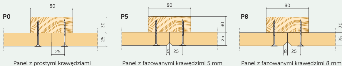
Panel z prostymi krawędziami
