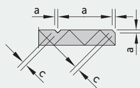
Kantenprofilabmessungen
