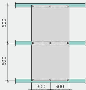
1200x600 mm paneli stiprināmi ar 9 skrūvēm.
