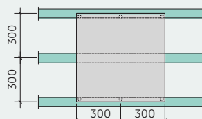
600x600 mm paneli stiprināmi ar 6 skrūvēm.
