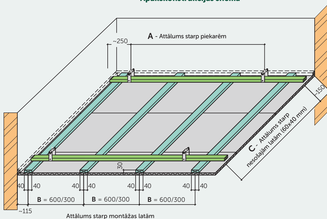
Apakškonstrukcijas shēma
