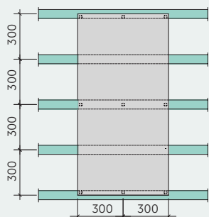
Panele 1200 x 600 mm: 9 wkrętów
