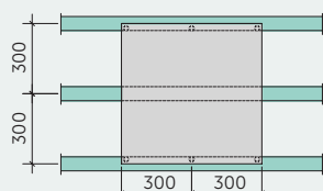
Panele 600 x 600 mm: 6 wkrętów
