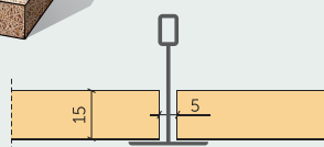
Plattendicke: 15 mm
