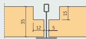
Plattendicke: 35 mm
