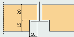
Plātnes biezums: 35 mm
