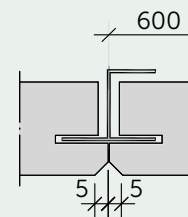
CEWOOD long edge profile P5H
