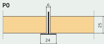
Einlegemontage in standard T-24-Profil
