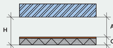
A – Luftspalt H – Gesamtkonstruktionshöhe C – CEWOOD FLEECE
