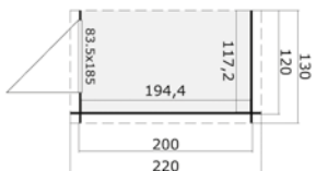
ARMOIRES JUXTAPOSABLES TOIT EN APPENTIS 200
