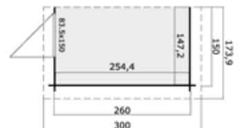
ARMOIRES JUXTAPOSABLES TOIT EN PIGNON 260
