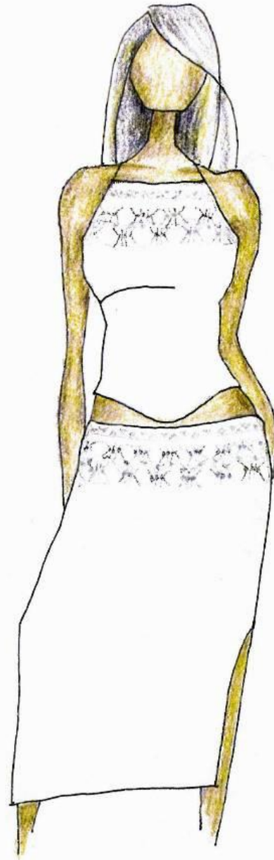
Mari Mardn
