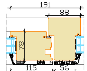
Transom
