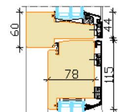
Transom
