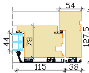
Standard jamb
