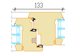
Avatav raam, püstimpost ja mitteavatav osa
