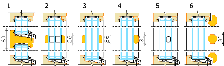
Standard jamb
