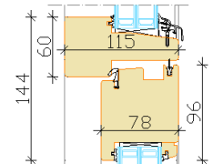
Transom
