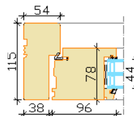
Standard jamb
