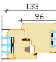
Avatav raam, püstimpost ja mitteavatav osa
