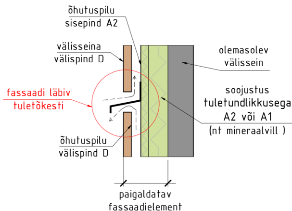
Joonis 2. Fassaadi läbiv tuletõkekesti
