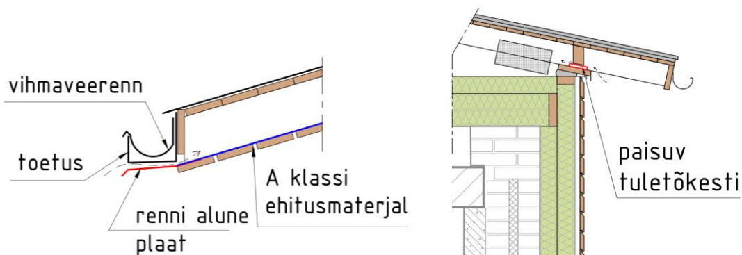
Joonis 2. Katuseräästa tuletõkestuse lahendamine
