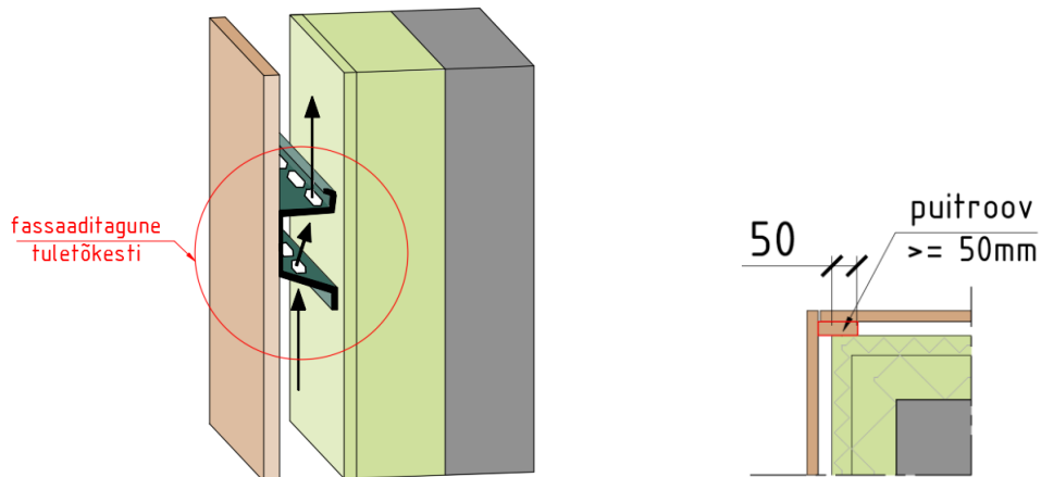
Joonis 3. Fassaaditagune tuletõkesti a) horisontaalne, tuulduv tuletõkesti b) vertikaalne, umbne tuletõkesti.
