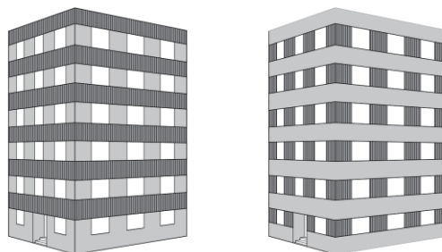
Joonis 9. Horisontaalne tulefõkestus kombineerituna põleva ja mittepõleva fassaadikatematerjaliga.
