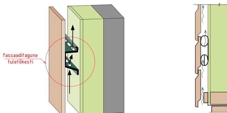
Joonis 10. Horisontaalse fassaadikatte taguse tulefõkesti lahendused. a) profileeritud metall; b) metallvõrguga loodud tulefõkesti jahutuse ja paisuva teibi ja õhuvoolu aeglustiga.
