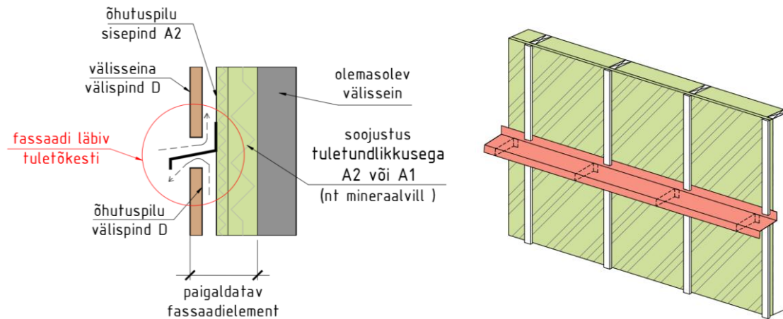
Joonis 11. (a) Horisontaalne tuletõkesti õhutuspilus ja (b) horisontaalse ja vertikaalse tuletõkesti paiknemine enne fassaadikatte paigaldust.
