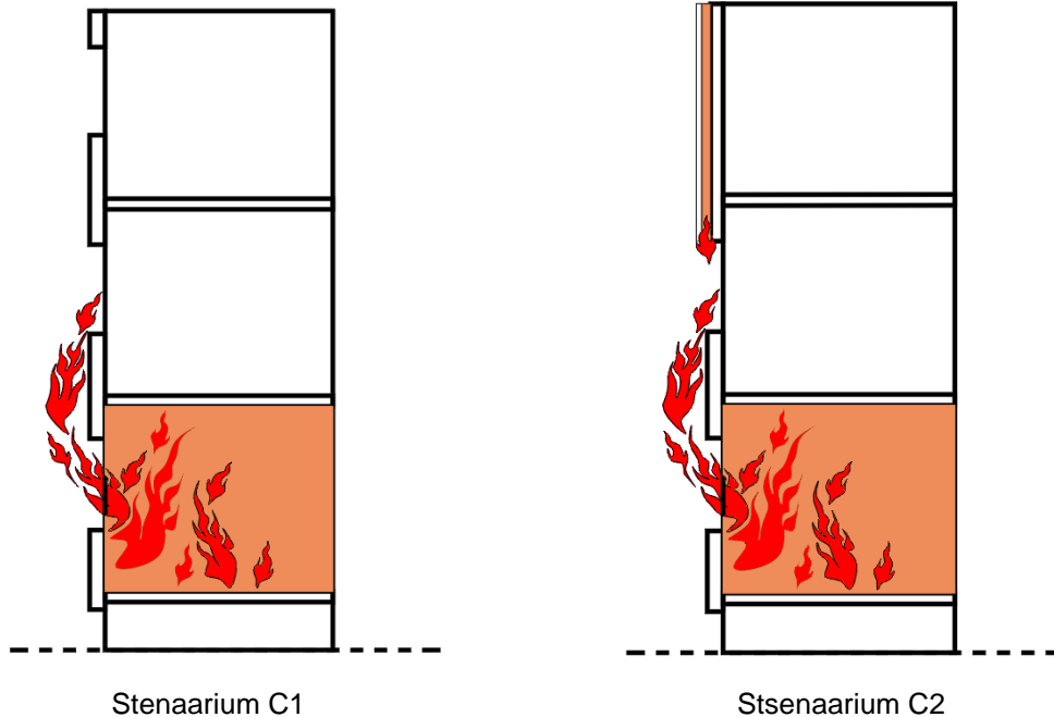
Joonis 5. Fassaadi tulekahju võib olla põhjustatud hoone sisese tulekahju poolt (C1). Tüheimikes võib tuli levida kiiremini ja kõrgemale (isegi 5-10 korda kõrgemale kui seda on väljaspool näha) kui seda on vaid otsese leegiga aknast(C2) 67 .
