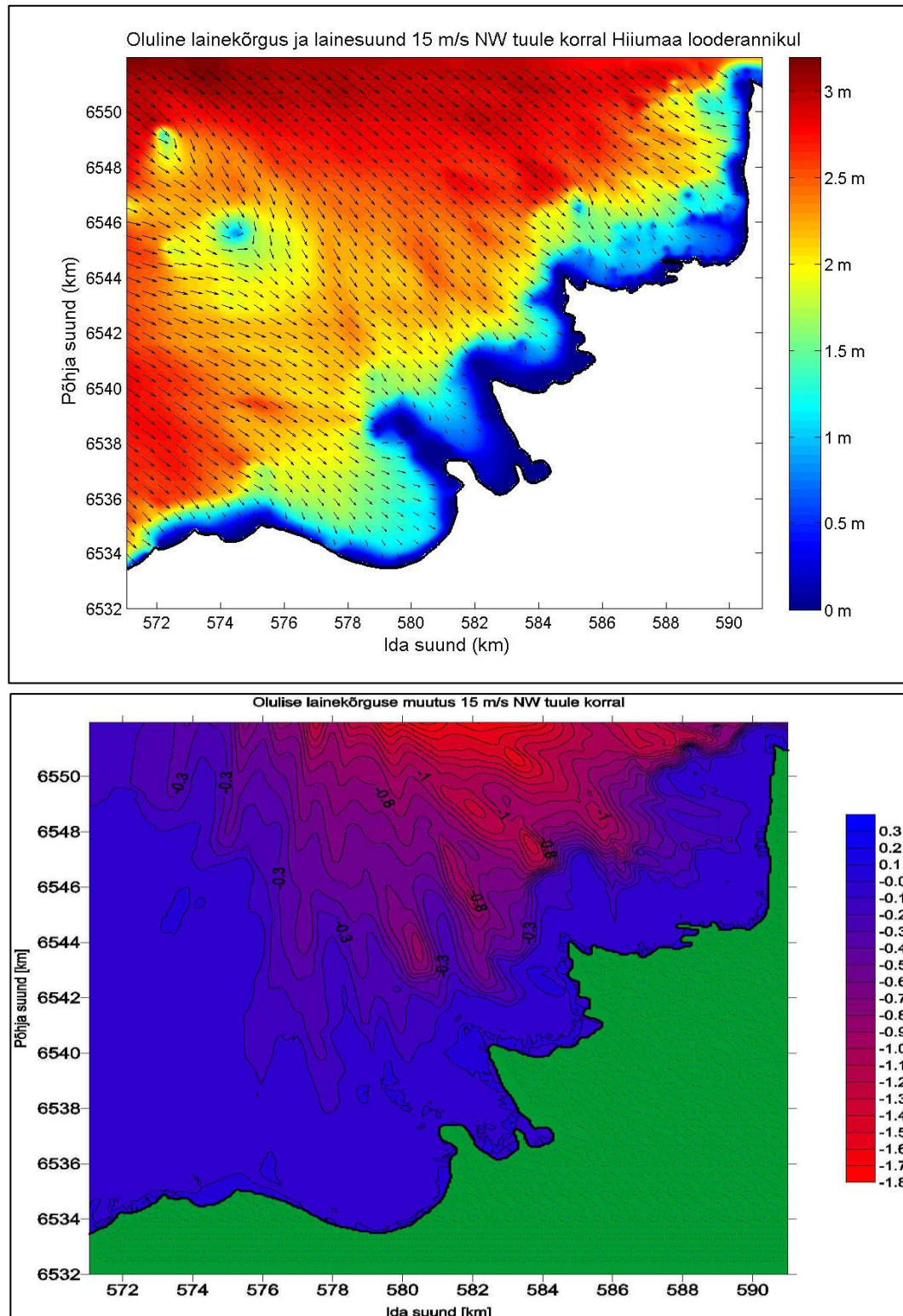
Joonis 141. Oluline lainekõrgus 15 m/s puhuva loodetuule korral (ülemine paneel) ja arendusalale TP 2 paigutatud tuulikute poolt põhjustatud olulise lainekõrguse muutus (cm, samuti 15 m/s puhuva loodetuule korral) Hiiumaa looderanniku lähistel (alumine paneel)
