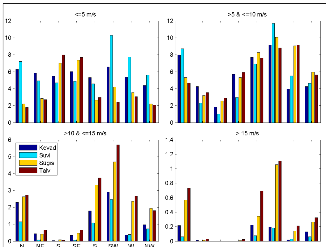
Joonis 28. Tuulte esinemissagedus (%) kevadel (märts-mai), suvel (juuni-august), sügisel (september-november) ja talvel (detsember-veebruar) jaotatuna nelja kiiruse ja kaheksasse suunavahemikku Vilsandil aastatel 1981-2012. Esinemissageduse telgede (vertikaaltelgede) skaalad varieeruvad
