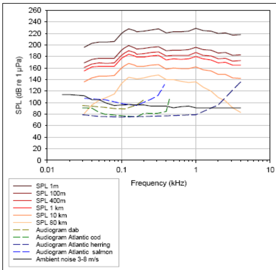
Joonis 158. Vaiade paigaldamise müra (ITAP 2005 järgi) nõrgenemine (ülevalt alla) erinevatel kaugustel allikast. Taustmüra DEWI (2004) järgi. Lisatud on ka kalade audiogrammid. X-teljel on indutseeritud heli sagedus kilohertsides. Y-teljel on toodud helirõhu tase detsibellides (Thomsen et al. 2006)
