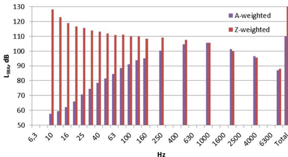
Joonis 165. 1/3 oktaavriba müratasemed Siemens SWT-4,0-130 elektrituulikudel
