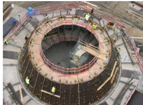
Joonis 8. Paigaldatud gravitatsioonvundament (325 MW avamere tuulepark Belgias)
