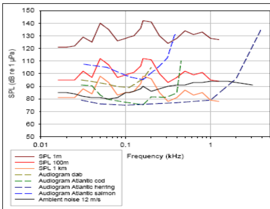
Joonis 159. Töömüra nõrgenemine (ülevalt alla) erinevatel kaugustel allikast. Töömüra arvutusel oli aluseks Rootsisis läbiviidud mõõtmine 1,5 MW tuulikuga (ITAP 2005). Lisatud on ka taustmüra väärtused (Betke et al. 2004) ning kalade audiogrammide (vt Joonis 158). Taustmüra mõõtmised viidi läbi Läänemeres tuulekiirusel 3 m/s (ITAP 2005). Need väärtused korrigeeriti kõrgemateks, sest tuulikute töö ajal on oodata kõrgemat tuule kiirust. X-teljel on indutseeritud heli sagedus kilohertsides. Y-teljel on toodud helirõhu tase detsibellides (Thomsen et al. 2006)
