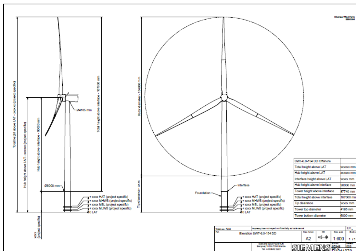
Joonis 6. Siemens SWT 6 MW tuuliku parameetrid
