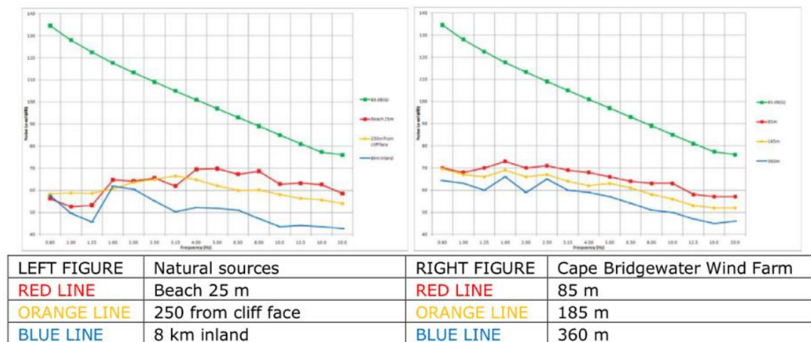
Joonis 163. Infraheli mõõtmistulemused erinevatel kaugustel tuulepargist 97
