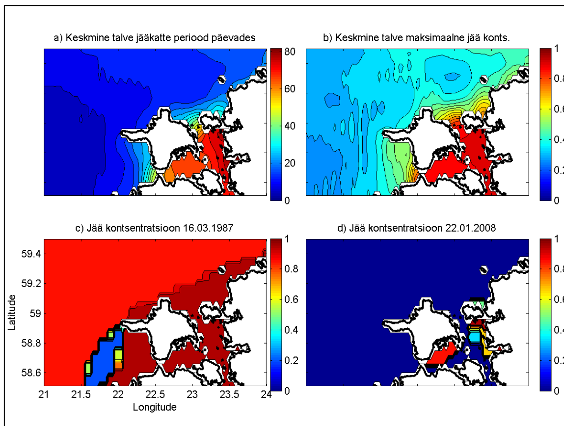
Joonis 31. Keskmine talve jääkatte periood päevades (a), keskmine talve maksimaalne jää kontsentratsioon 1982-2009 (b) ning jää kontsentratsioon 16.03.1987 (c) ja jää kontsentratsioon 22.01.2008 (d) Hiiumaa lähisel. Joonise tegemisel on kasutatud Taani Meteoroloogia Instituudi poolt satelliitseire põhjal koostatud Läänemere jääolude andmebaasi
