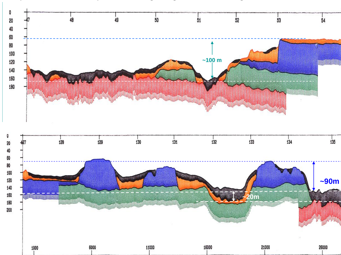
Joonis 22. Ülemine profiil loode-kagu suunaline ja alumine profiil kirde-edela suunaline geoloogiline läbilõige Balti klindi veeluse osa servaalast rahvusvahelistes vetes Hiiumaast ca 15-20 km läänes (K. Orviku ja B. Winterhalter'i poolt interpreteeritud seismo-akustilise pidevsondeerimise läbilõiked, käsikiri)
