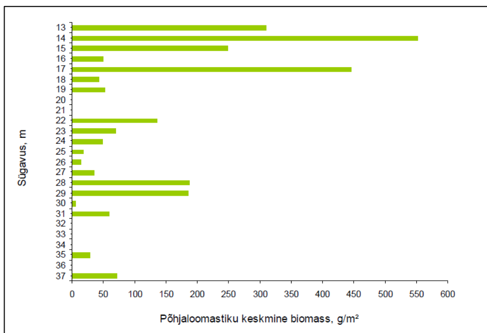
Joonis 82. Inventuuri aladel esinevad põhjajoomastiku keskmised biomassid (g/m²) vastavalt sügavuslevikule (m). Andmed ainult nendest proovipunktidest, kus esines põhjajoomestikku
