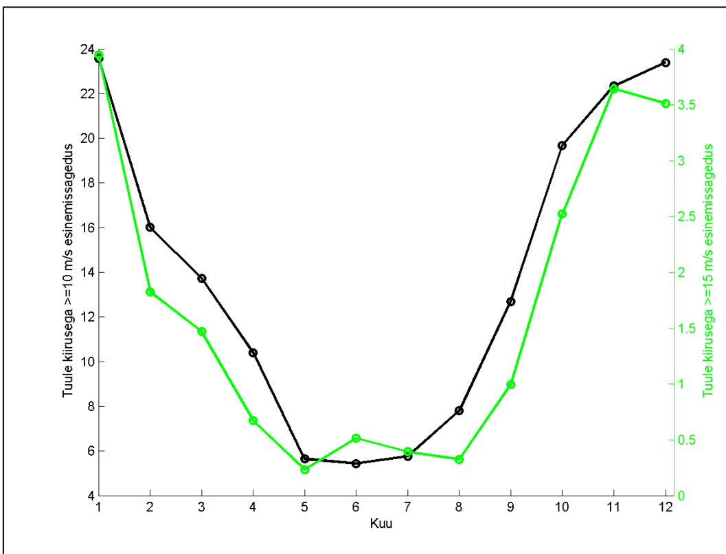
Joonis 27. Keskised \geq 10 m/s ja \geq 15 m/s tuule esinemissagedused (%) kuude kaupa Vilsandil aastatel 1981-2012
