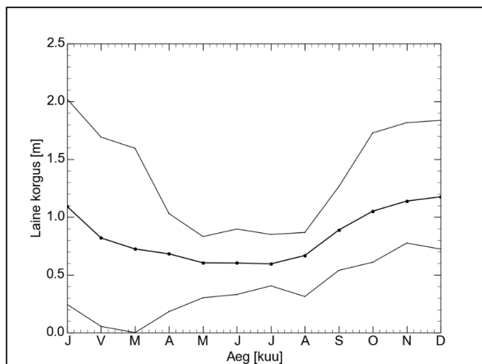
Joonis 48. Modelleeritud kuu keskmise olulise lainekõrguse aastane käik (keskmine joon) koos kuu keskmise olulise lainekõrguse minimaalse ja maksimaalse väärtusega aastatel 1965-2005 madaliku neljas piirkonnas
