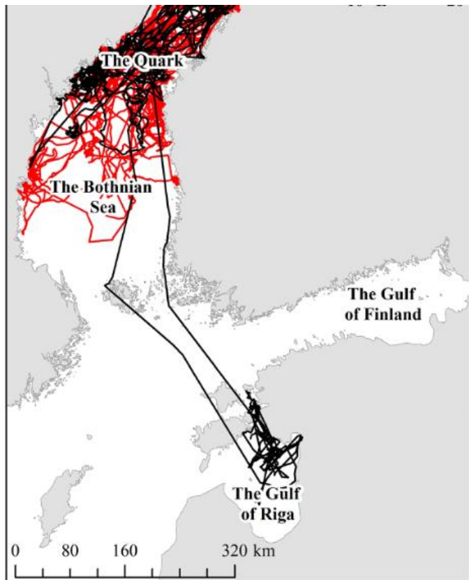
Joonis 112. Märgistatud viiherhüljeste ränded Läbi tuulepargi alade piirkonna (Oksanen jt 2015).
