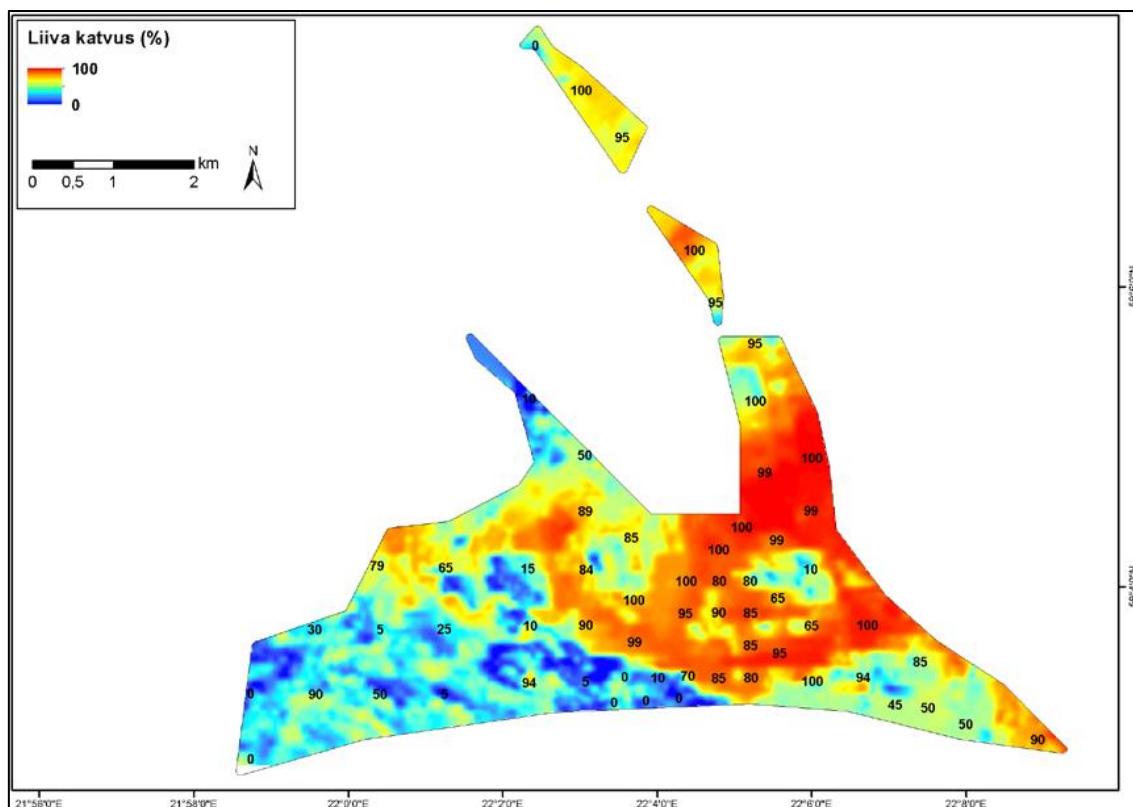
Joonis 69. Arendusala TP 4 uuritud ala liiva katvus (%). Lisaks modelleerimistulemustele on kaardil ära toodud numbritena jaamade videomaterjali analüüsi käigus saadud kõva põhjasubstraadi katvus (%)
