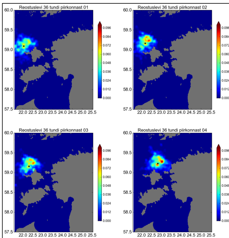
Joonis 175. Reostuslevi tõenäosus 36 h jooksul erinevatest tuuleparkide asukohtadest 2012. aastal
