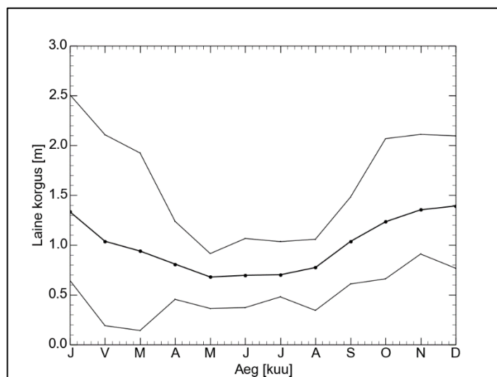
Joonis 45. Modelleeritud kuu keskmise olulise lainekõrguse aastane käik (keskmine joon) koos kuu keskmise olulise lainekõrguse minimaalse ja maksimaalse väärtusega aastatel 1965–2005 madaliku ühes piirkonnas
