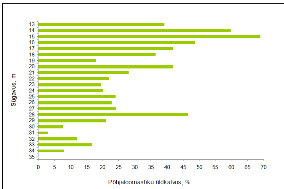
Joonis 83. Inventuuri aladel esinevad põhjajoomastiku keskmised katvused (%) vastavalt sügavuslevikule (m). Sügavustel 35 m on keskmine biomass 0.1 g/m² ning sellest tulenevalt ei kajastu see joonisel. Andmed ainult nendest proovipunktidest, kus esines põhjajoomestikku
