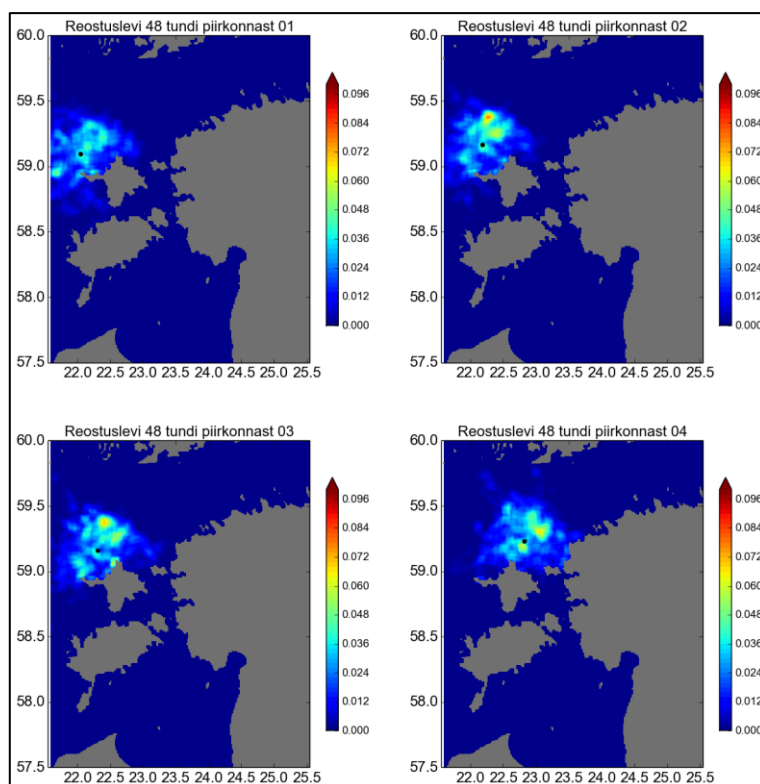
Joonis 177. Reostuslevi tõenäosus 48 h jooksul erinevatest tuuleparkide asukohtadest 2012. aastal
