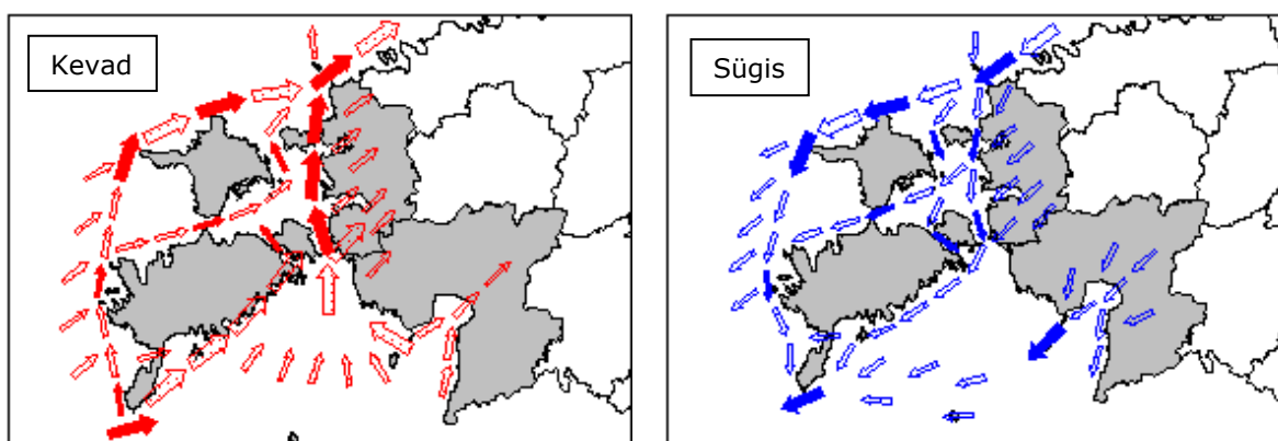
Joonis 160. Arktiliste veelindude transiitränne Lääne-Eesti rannikualal
