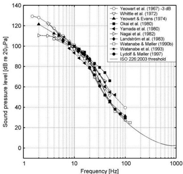
Joonis 162. Infraheli tajumislävi 90
