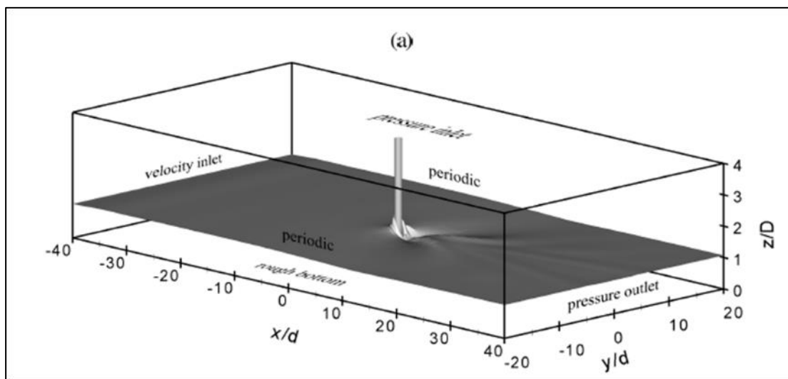
Joonis 149. Vette paigutatud tuuliku jala mõju modelleerimise skeem (Rennau, 2011).
