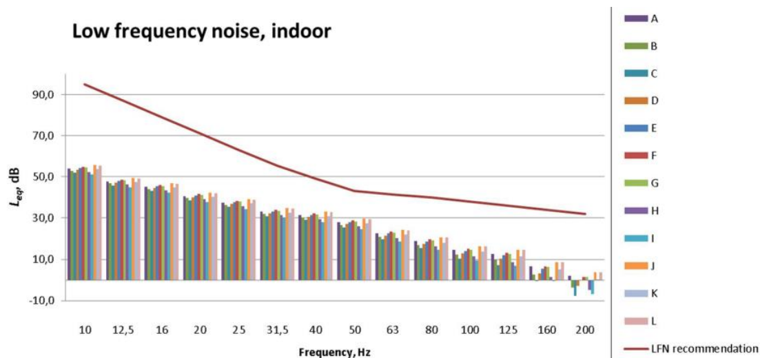
Joonis 166. 1/3 oktaavriba madalsagedusliku müra tase vastuvõtupunktides hoonetes sees
