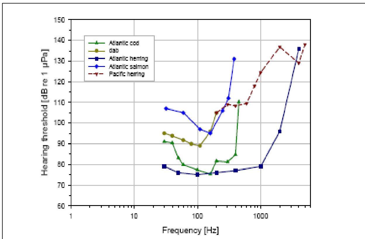
Joonis 157. Audiogrammid liikidele Atlandi lõhe ( Atlantic salmon ) (Hawkins & Johnstone 1978), Atlandi tursk ( Atlantic cod ) (Chapman & Hawkins 1973), Atlandi heeringas ( Atlantic herring ) (Enger 1967) ja soomuslest ( dab ) (Chapman & Sand 1974). Võrdlusemomendi tekitamiseks on lisatud veel Vaikse ookeani heeringas ( Pacific herring , Clupea pallasii ), kes on tuntetu ultrahelile (Mann et al. 2005). X-teljel on indutseeritud heli sagedus hertsides. Y-teljel on toodud kuulmislävi detsibellides (Effects of offshore wind farm noise on marine mammals and fish, 2006)
