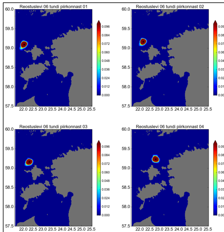
Joonis 171. Reostuslevi tõenäosus 6 h jooksul erinevatest tuuleparkide asukohtadest 2012. aastal
