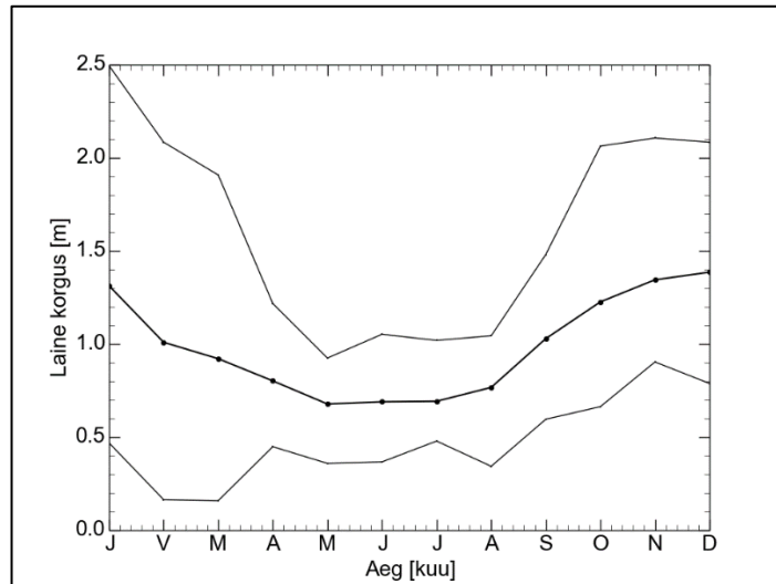
Joonis 46. Modelleeritud kuu keskmise olulise lainekõrguse aastane käik (keskmine joon) koos kuu keskmise olulise lainekõrguse minimaalse ja maksimaalse väärtusega aastatel 1965-2005 madaliku kahes piirkonnas
