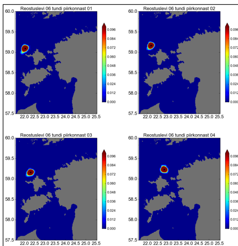
Joonis 170. Reostuslevi tõenäosus 6 h jooksul erinevatest tuuleparkide asukohtadest 2011. aastal. Must täpp on algallika asukoht
