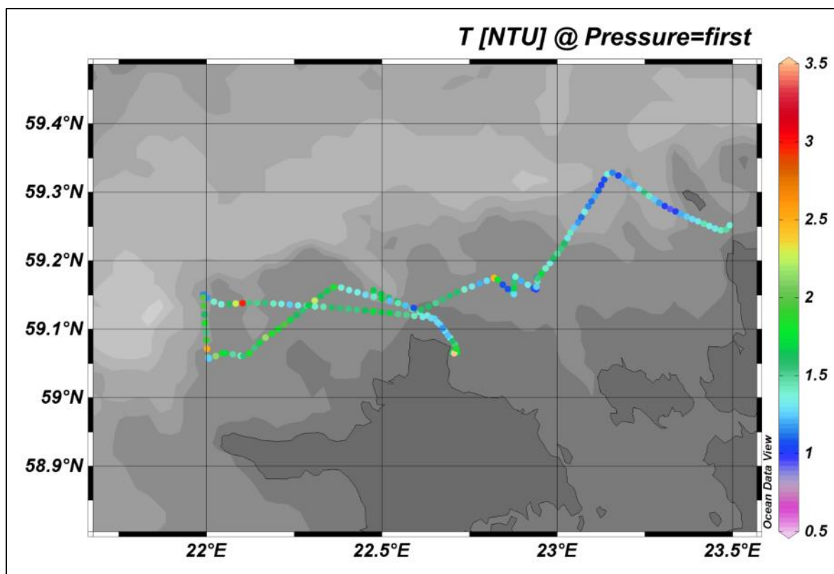
Joonis 36. Uurimislaeva SALME läbivoolusüsteemiga mõõdetud vee hägusus (NTU) Hiiumaa madalate piirkonnas 29.04.2014
