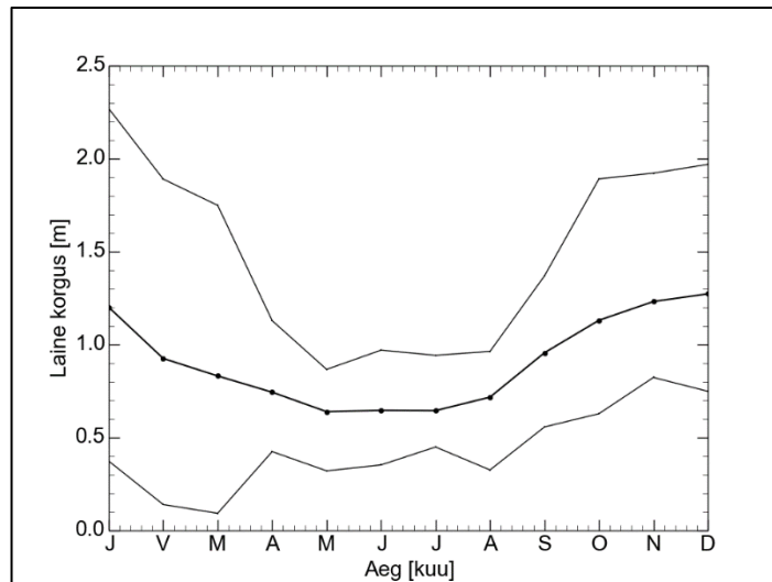
Joonis 47. Modelleeritud kuu keskmise olulise lainekõrguse aastane käik (keskmine joon) koos kuu keskmise olulise lainekõrguse minimaalse ja maksimaalse väärtusega aastatel 1965-2005 madaliku kolmes piirkonnas
