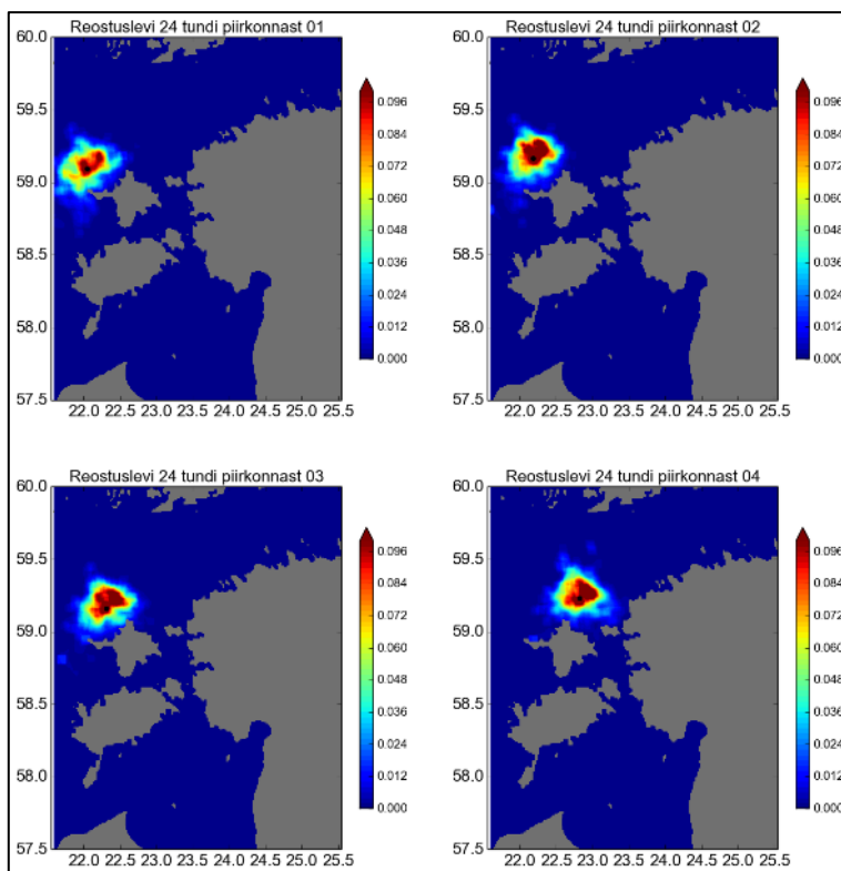
Joonis 173. Reostuslevi tõenäosus 24 h jooksul erinevatest tuuleparkide asukohtadest 2012. aastal
