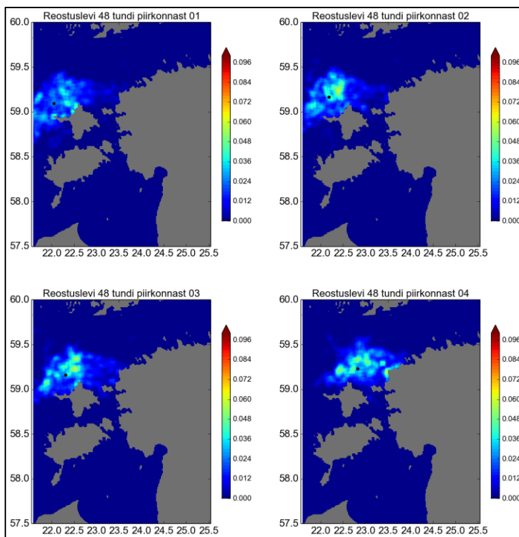
Joonis 176. Reostuslevi tõenäosus 48 h jooksul erinevatest tuuleparkide asukohtadest 2011. aastal
