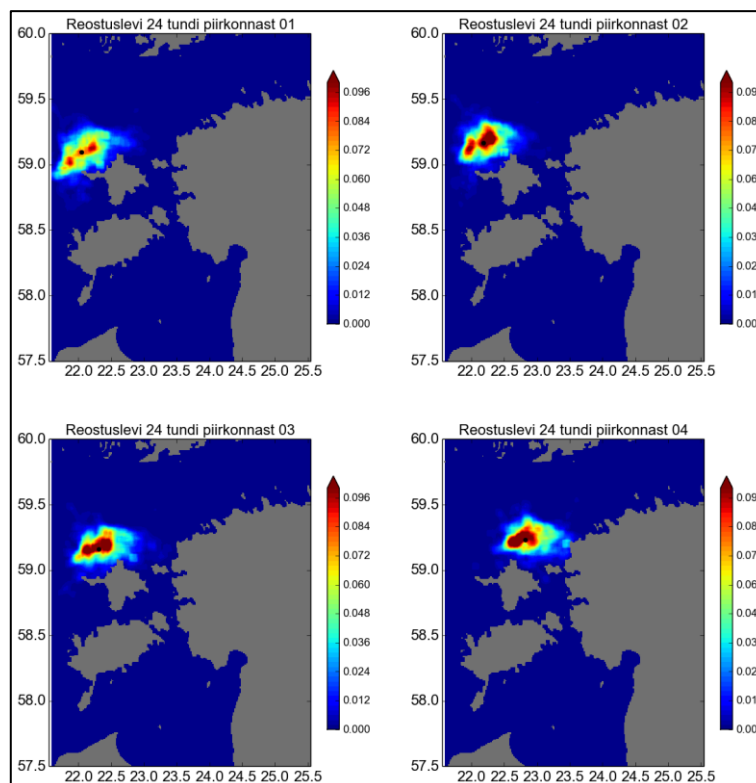
Joonis 172. Reostuslevi tõenäosus 24 h jooksul erinevatest tuuleparkide asukohtadest 2011. aastal
