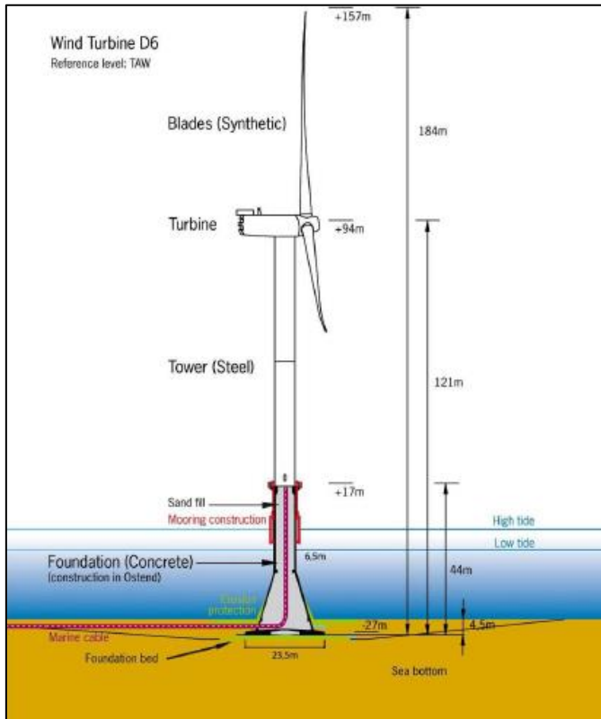
Joonis 8. Paigaldatud gravitatsioonvundament (325 MW avamere tuulepark Belgias)
