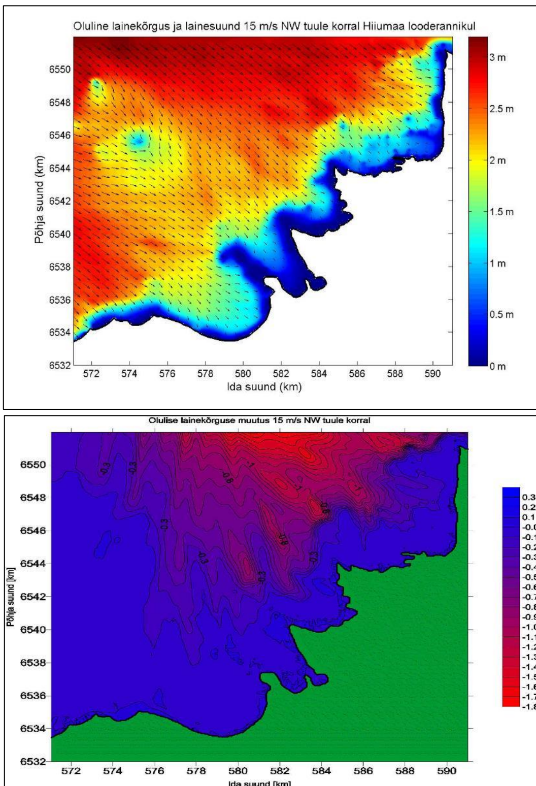
Joonis 148. Oluline lainekõrgus 15 m/s puhuva loodetuule korral (ülemine paneel) ja arendusalale TP 2 paigutatud tuulikute poolt põhjustatud olulise lainekõrguse muutus (cm, samuti 15 m/s puhuva loodetuule korral) Hiiumaa looderanniku lähistel (alumine paneel)
