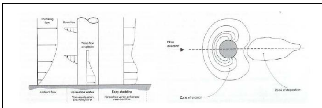
Joonis 150. Pinnase erosioon ja täiskandumine püsivast suunast liikuva hoovuse ja toruja tuuliku vastasmõju tagajärjel (Whitehouse, R, 1998)
