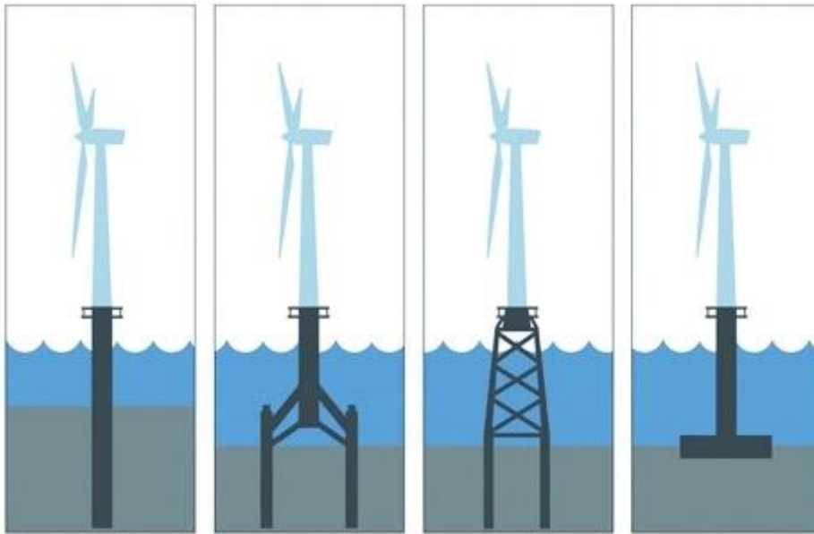
Joonis 7. Elekrituuliku vundamentide tüübid (vasakult: vai-, kolmjalg-, sõrestik ja gravitatsiooni-vundament) 3
