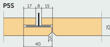
Slēptais piekārtu griestu profils ar pārkari un 5 mm fāzi
