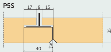
Slēptais piekārtu griestu profils ar pārkari un 5 mm fāzi
