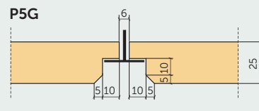
legremdēts T24 griestu profils ar 5 mm fāzi
