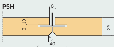
Slēptais piekārtu griestu profils ar 5 mm fāzi
