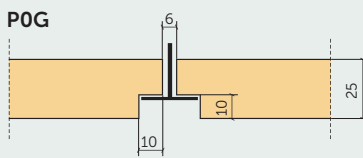
legremdēts T24 griestu profils
