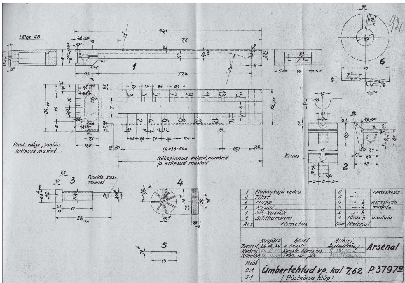
Arsenali kaasaegne sektorsihik kütipüssile. (ERA)
