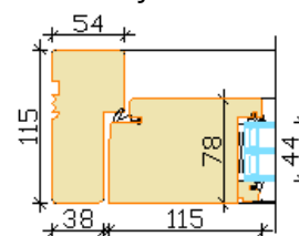
Standard jamb
