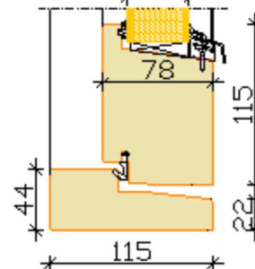
Standard jamb
