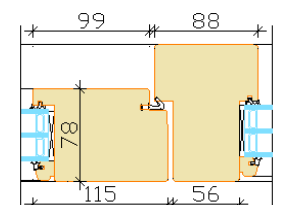
Transom
