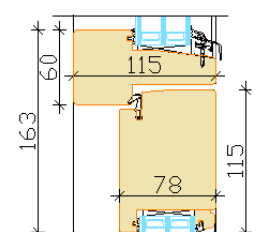
Transom
