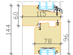
Rõhtipost
